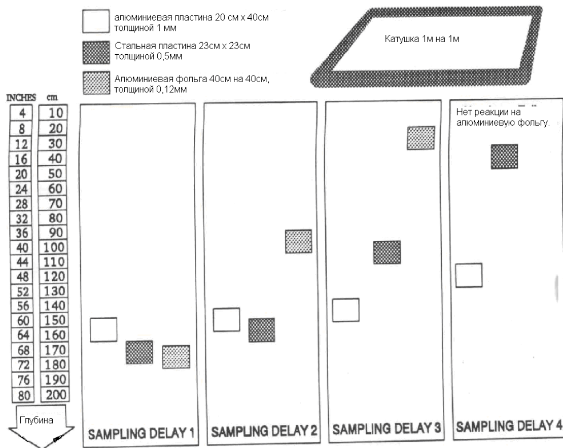
Рис.6. Зависимость глубины поиска от положения переключателя SAMPLING DELAY.
